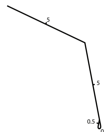
26. GAMBREL TRIM
