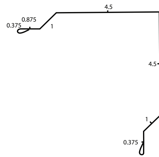
2. RAKE & CORNER
