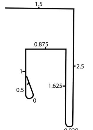
20. C&T CHANNEL
